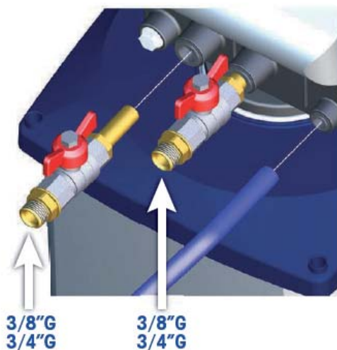
Detail pripojenia
